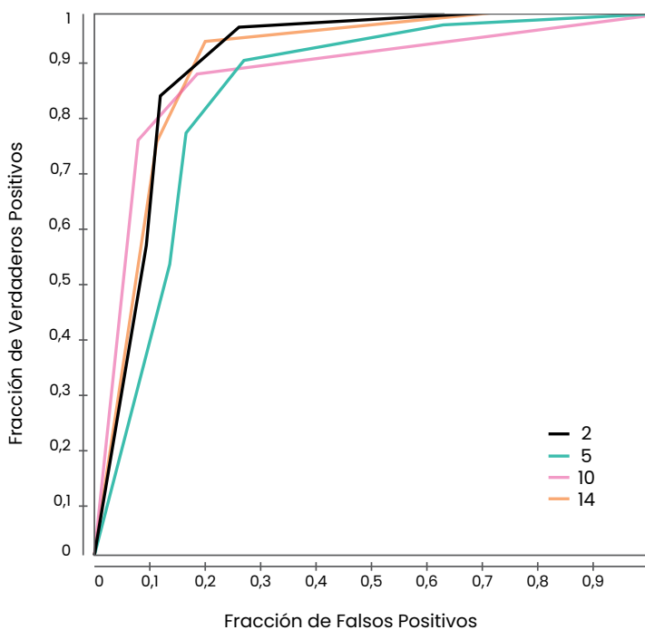
Curvas de características operativas del receptor (ROC) para diferentes corrientes de tubo (2, 5, 10, 14 mA)
